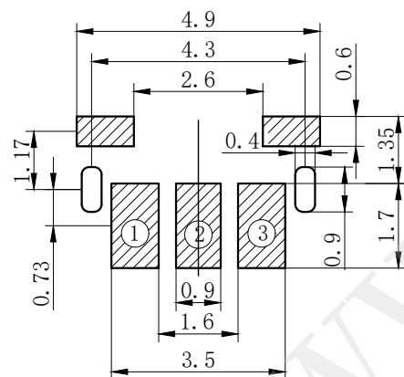
安装参考图
